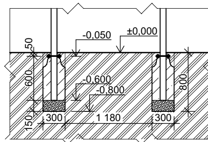
KOTVENÍ ZALITÍM
